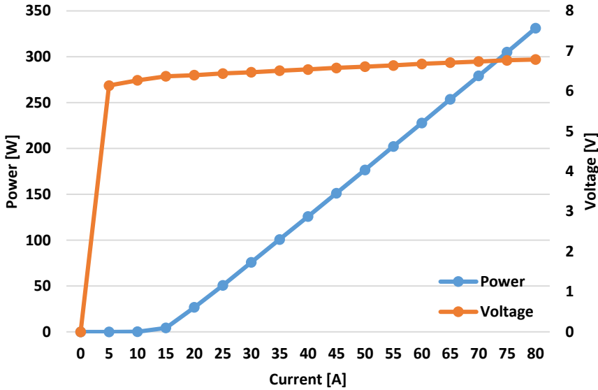
L-I-V Characteristics
